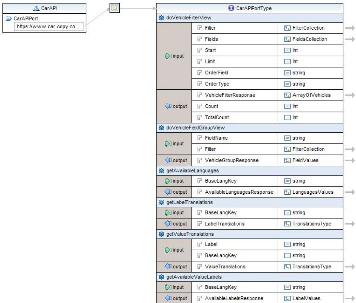
Abbildung 3.1: WSDL Schema
